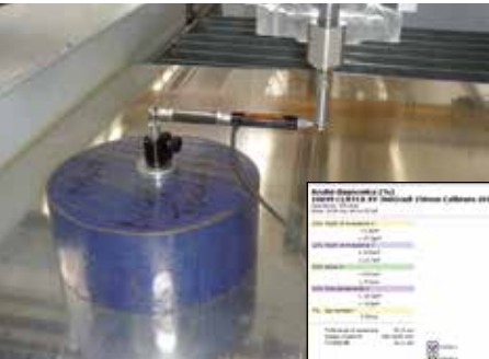
Renishaw Ball Bar inspection and verification Controllo circolarità con Ball Bar Renishaw
