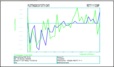
Renishaw Laser Straightness and Linearity control and compensation Controllo e Compensazione di Rettilinearità e Linearità tramite Laser Renishaw
