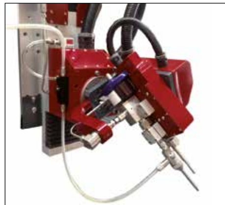
Edge 5 axis ±55° interpolating system up to 4.150 Bar with I.T.C.™ (Intelligent Tapering Control) Sistema Edge a 5 assi interpolanti ±55° fino a 4.150 Bar con I.T.C.™ (Compensazione Conicità)
