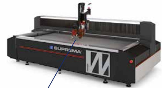
Edge 5™ 5 AXIS ±55° (Optional)
